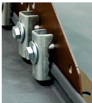
Кронштейн на двойном стоячем фальце (без затяжки)
