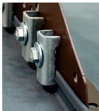
Кронштейн на двойном стоячем фальце (с затяжкой)
